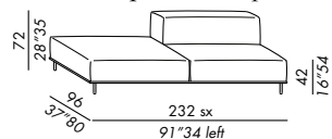
elemento penisola - penisula unit 235
