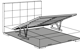
storage box profondità - depth cm. 18 - 7 1/8
