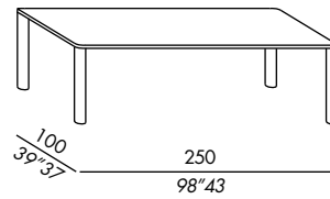
tavolo pranzo / dining table TP-250100
