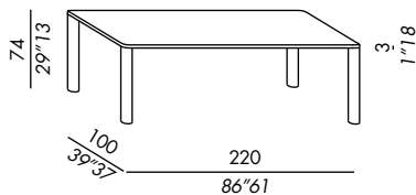
tavolo pranzo / dining table TP-220100
